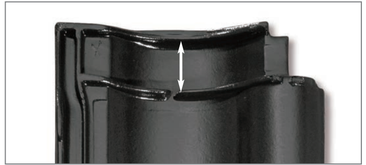
Extragroße Verschiebemöglichkeit, bis zu 25 mm Höhenüberdeckung
