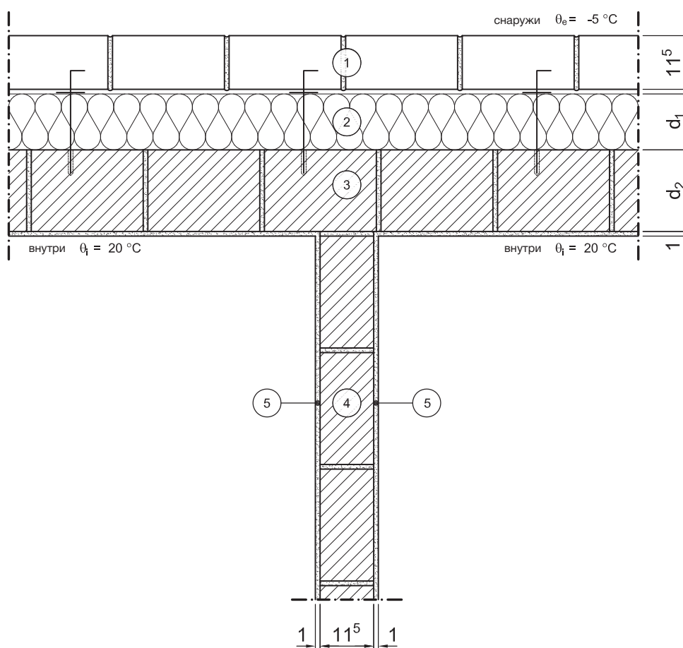
Горизонтальный разрез
