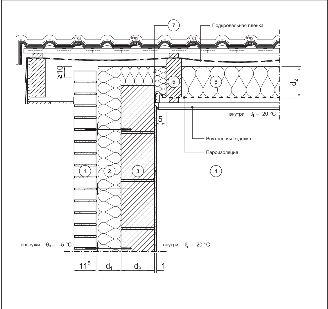
Вертикальный разрез Масштаб 1:10
