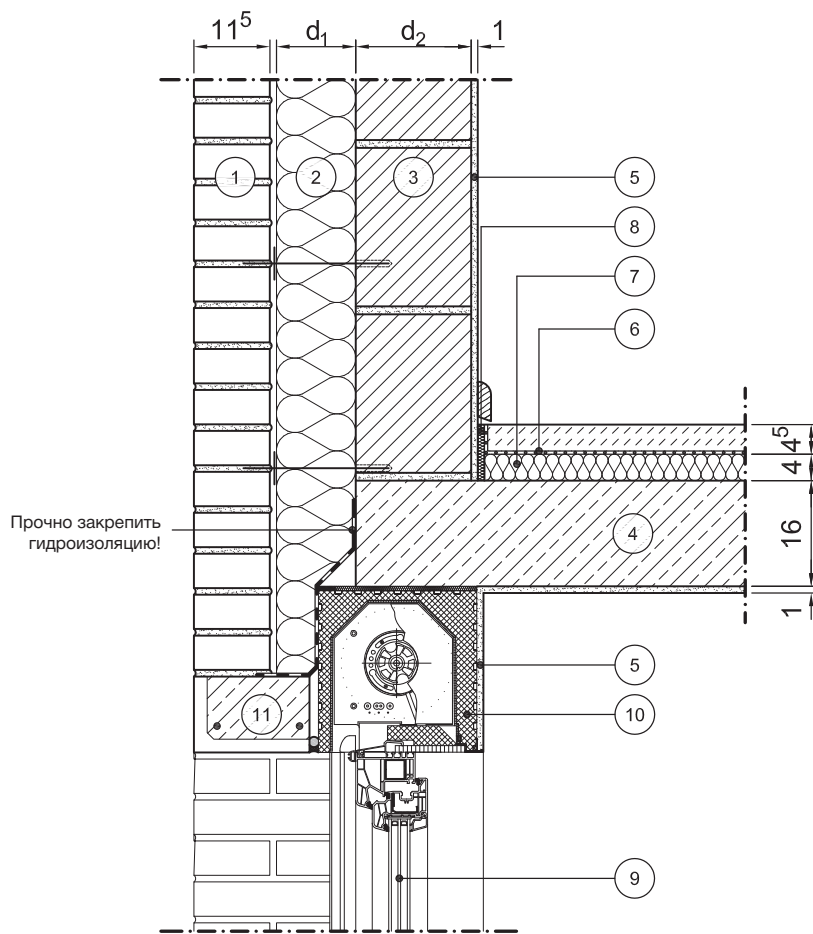
Вертикальный разрез
