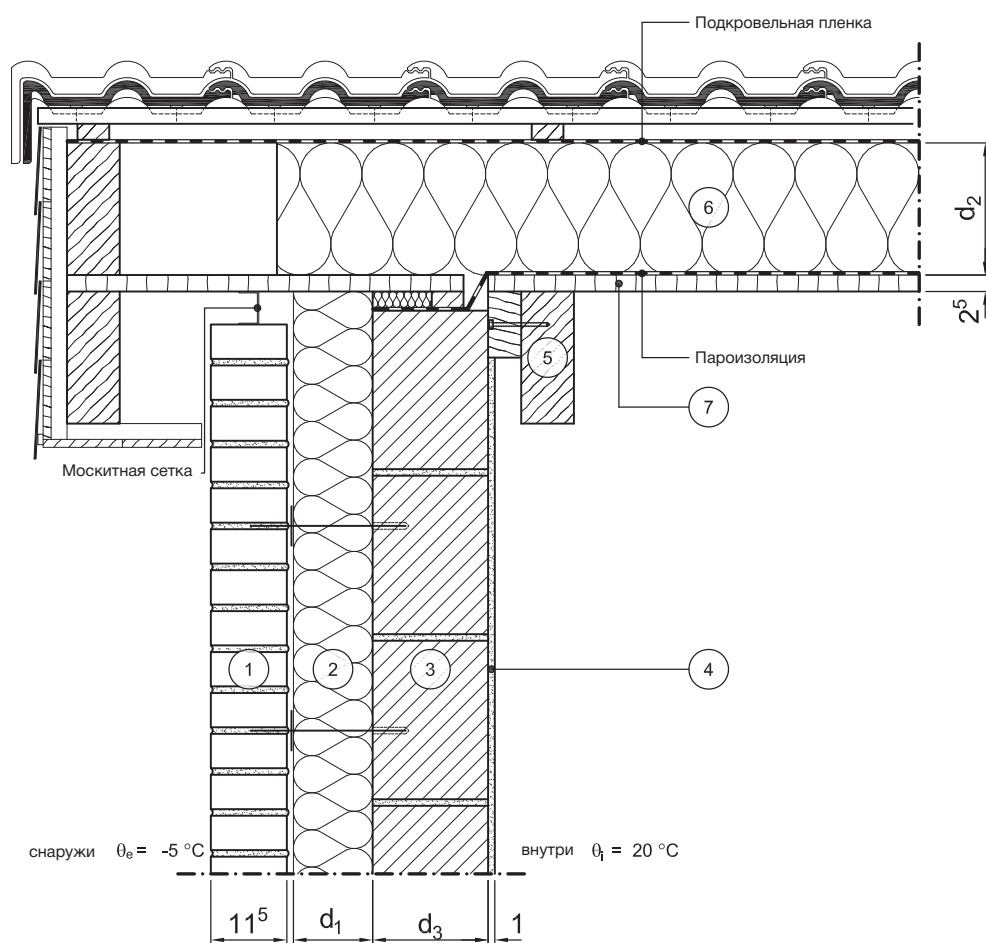
Вертикальный разрез
