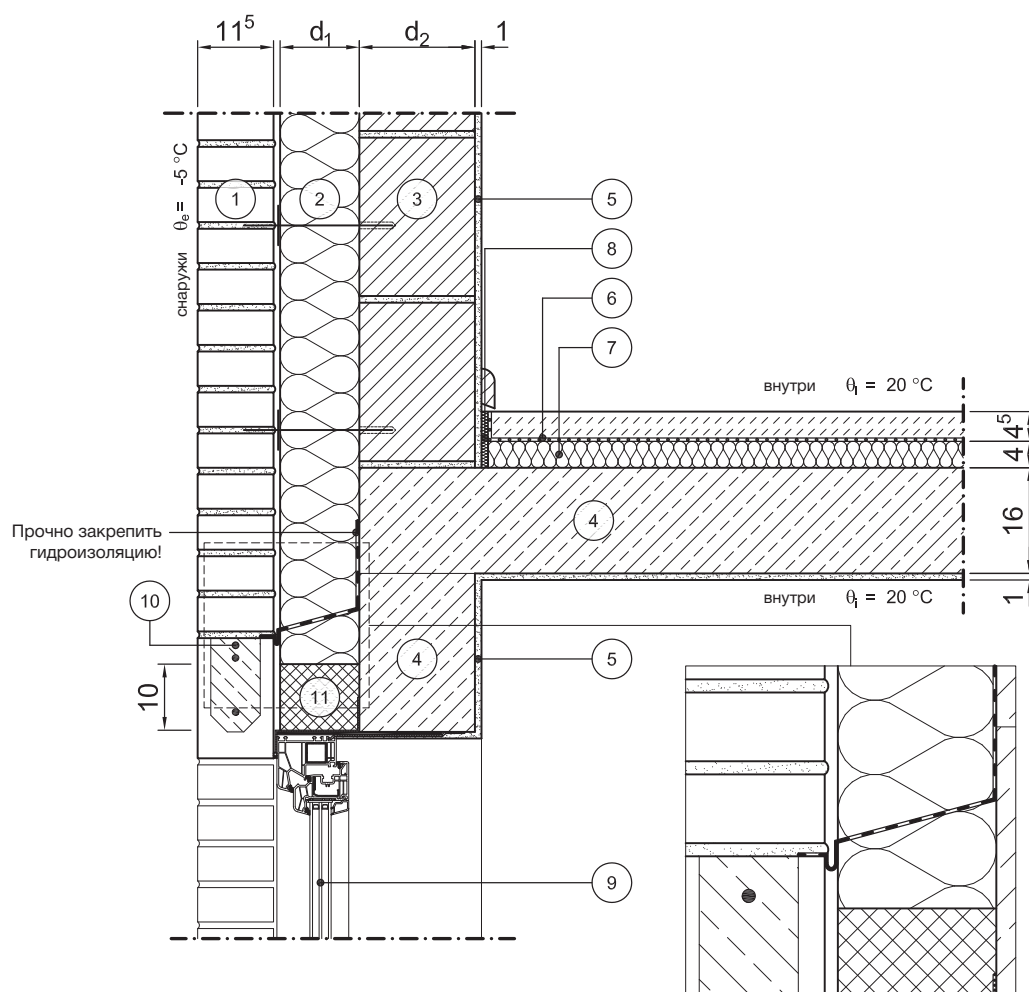
Вертикальный разрез
