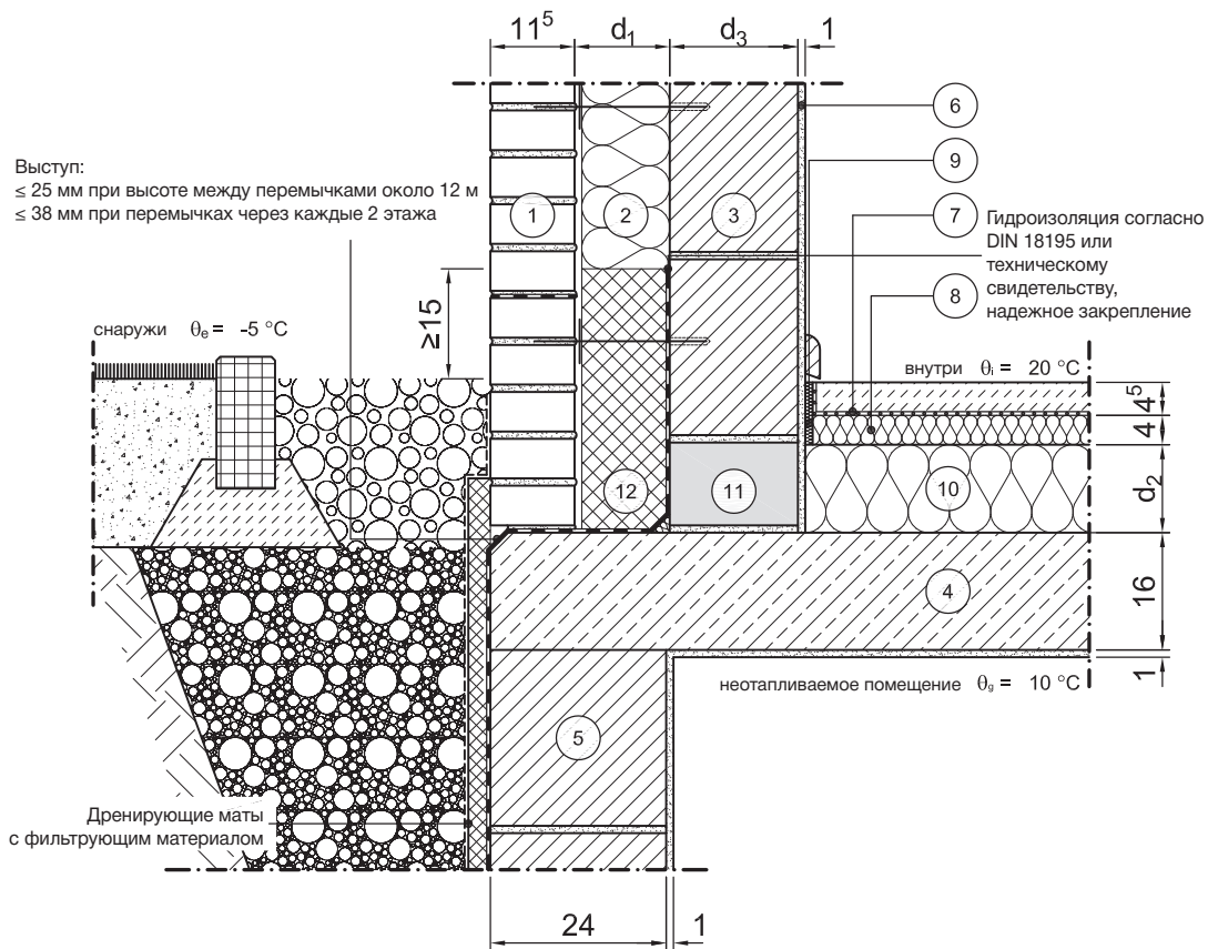
Вертикальный разрез
