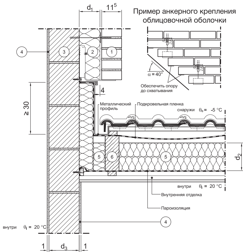
Вертикальный разрез Масштаб 1:10
